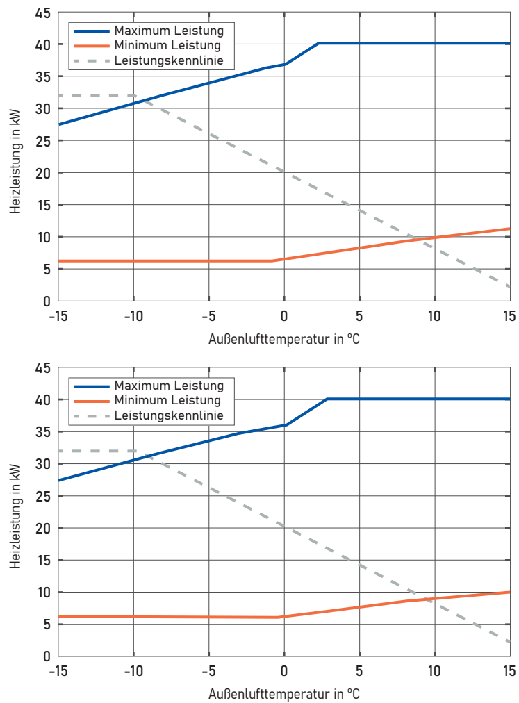
Abb. 9: Leistungsbereich der EU35L je nach Außenlufttemperatur bei 5K Spreizung und 85 % Luftfeuchte (oben: 35 °C Vorlauftemperatur / unten: 55 °C Vorlauftemperatur) mit empfohlener Leistungskennlinie nach EN 14825.
