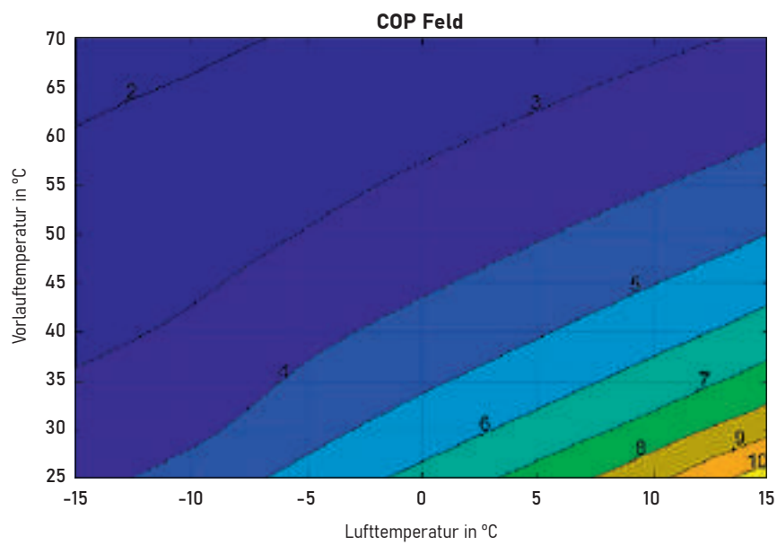
Abb. 10: EU35L bei 20kW Heizleistung
